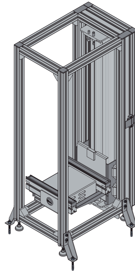
昇降リフト
